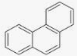
fenantreno
